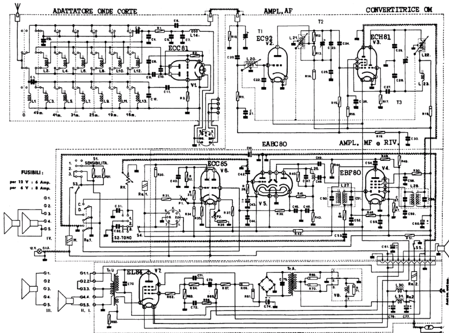
I S. A. - Autoradio PHONOLA-BECKER mod. 731. Apparecchio con ricerca automatica delle emittenti, ottenuta con dispositivo elettronico (V5 e V6); l'indice si ferma sui trattini rispondenti a stazioni ricevibili con tre gradi di sensibilità dell'apparecchio. Dispositivo per il comando a distanza. Adattatore per onde corte. Sintonia a permeabilità variabile. (V. retro caratteristiche e note di servizio).
